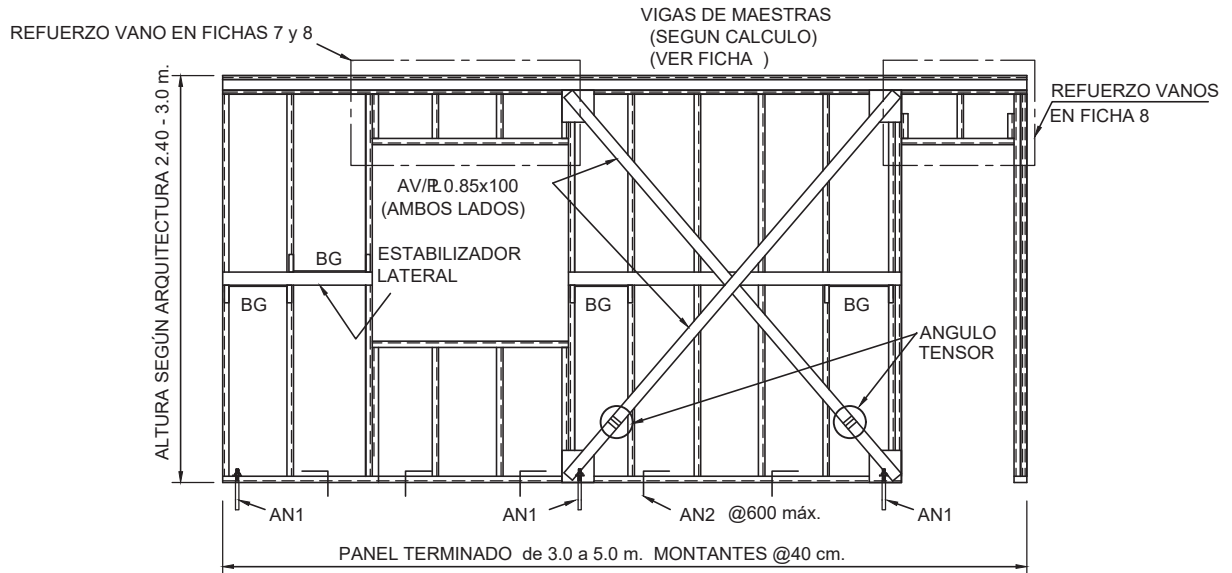
ELEVACION TIPICA MURO MP2
